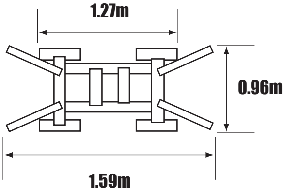
クレーン台車寸法
