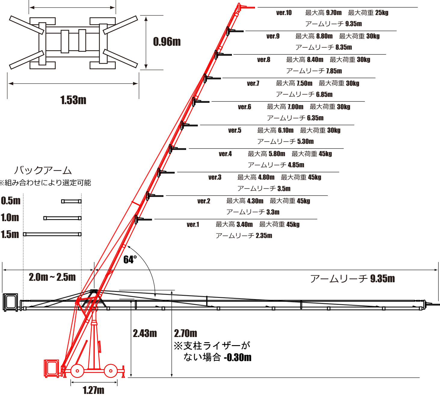
クレーン台車寸法
