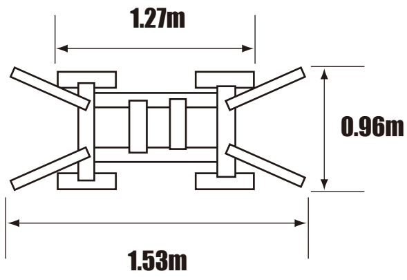
クレーン台車寸法
